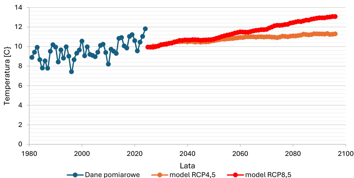
Wykres 31 Zmienność i prognozowane trendy zmian średniej rocznej temperatury powietrza w Opolu 47,48
