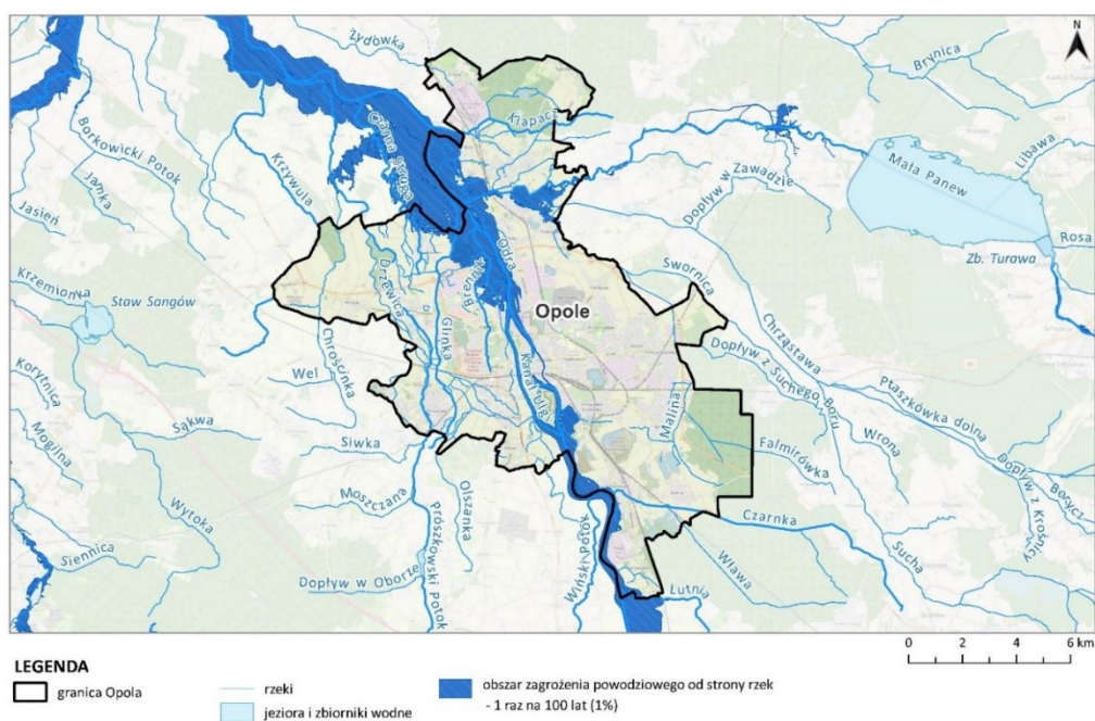
Rysunek 22 Obszary zagrożenia powodziowego 1% w zasięgu Opola 85
