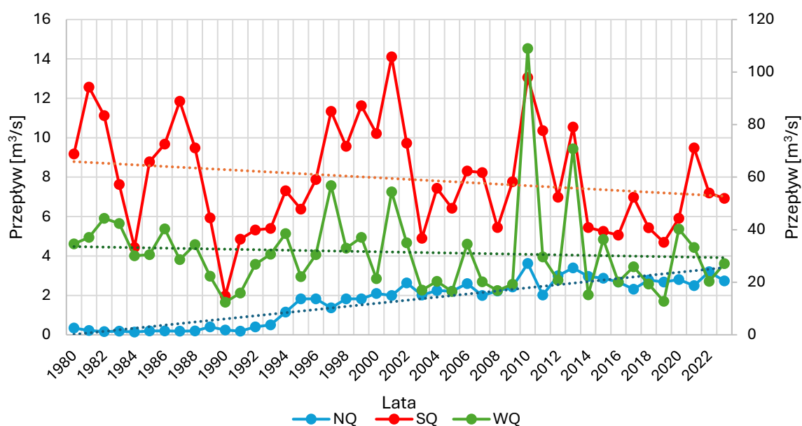
Wykres 25 Przebieg wartości NQ, SQ oraz WQ dla posterunku wodowskazowego Turawa 27
