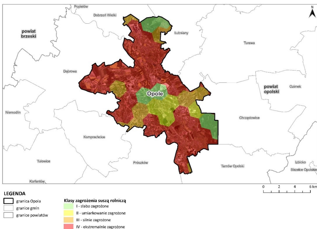
Rysunek 26 Zagrożenie suszą rolniczą w zasięgu Opola 92
