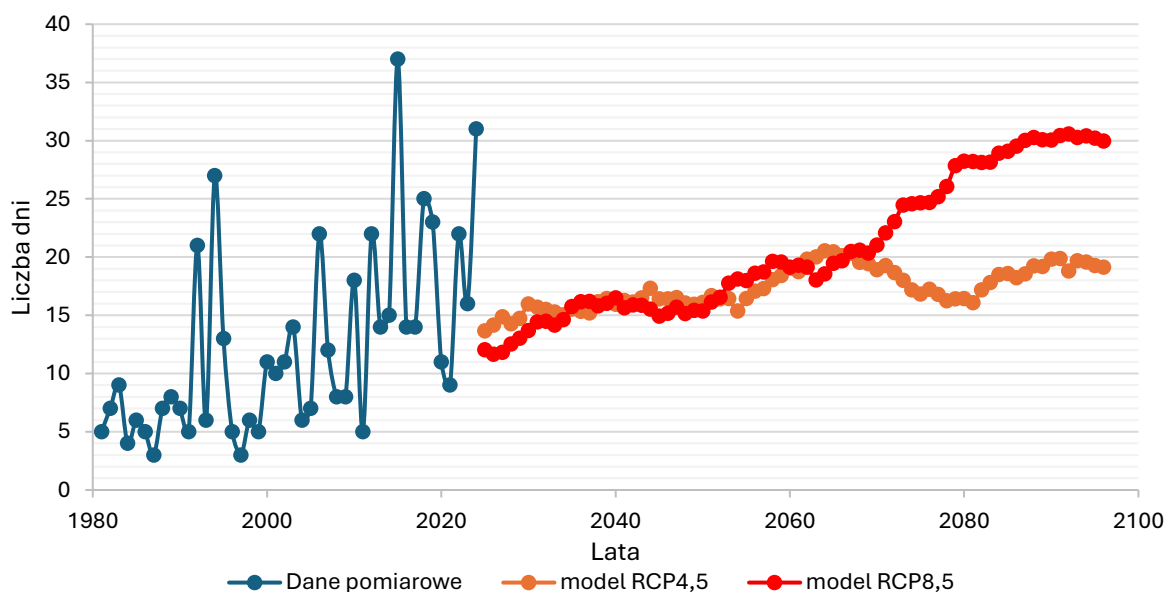
Wykres 32 Zmienność i prognozowane trendy zmian liczby dni upalnych w Opolu 49,50
