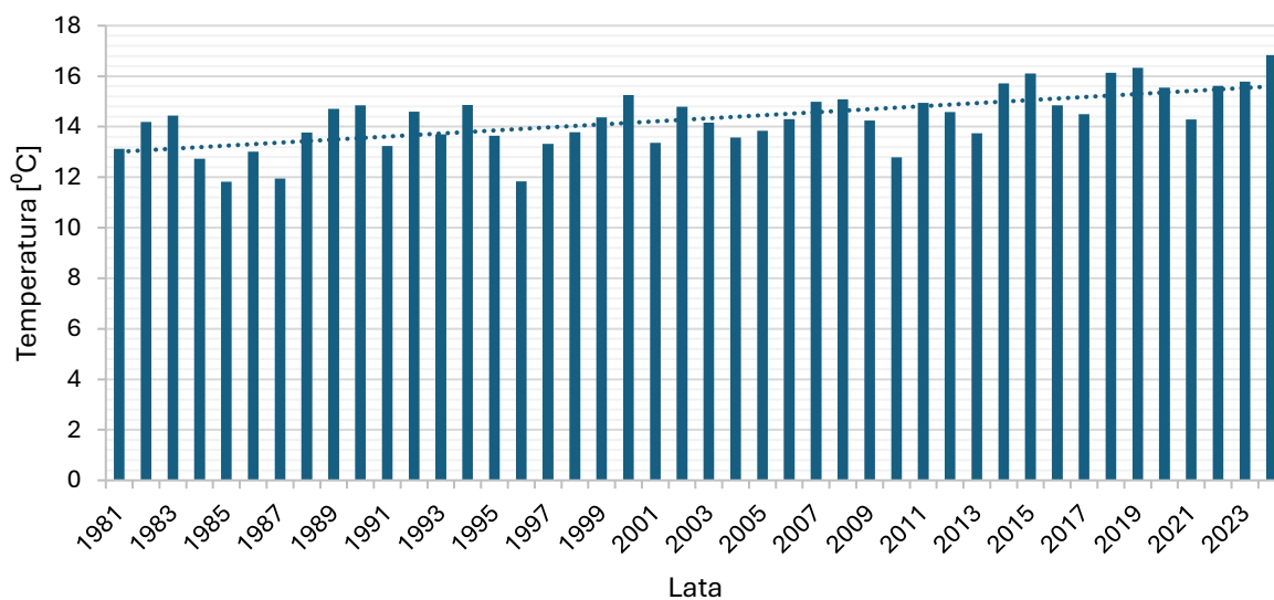
Wykres 3 Przebieg średnich wartości temperatury maksymalnej powietrza w Opolu 3
