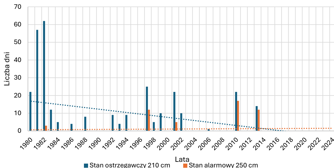
Wykres 26 Liczba wystąpienia w poszczególnych latach stanów ostrzegawczych i alarmowych dla posterunku wodowskazowego Turawa 28
