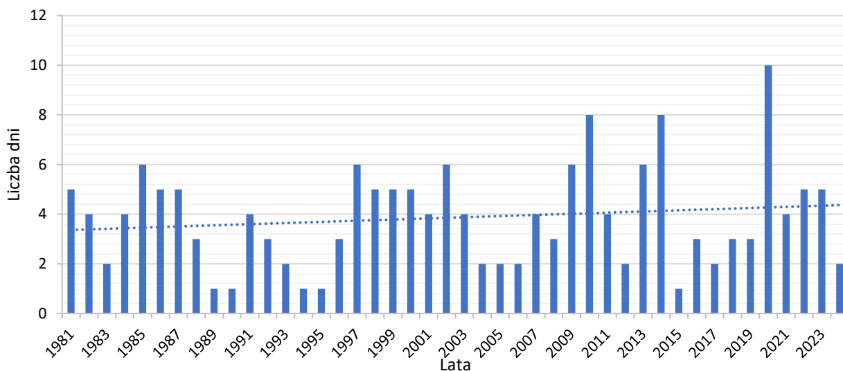
Wykres 4 Częstość występowania opadów atmosferycznych o sumie dobowej co najmniej 20 mm w Opolu 4
