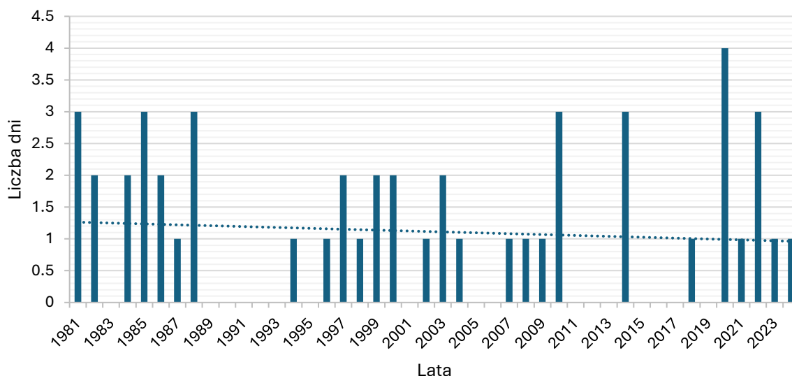
Wykres 19 Częstość występowania opadów atmosferycznych o sumie dobowej co najmniej 30 mm w Opolu 20
