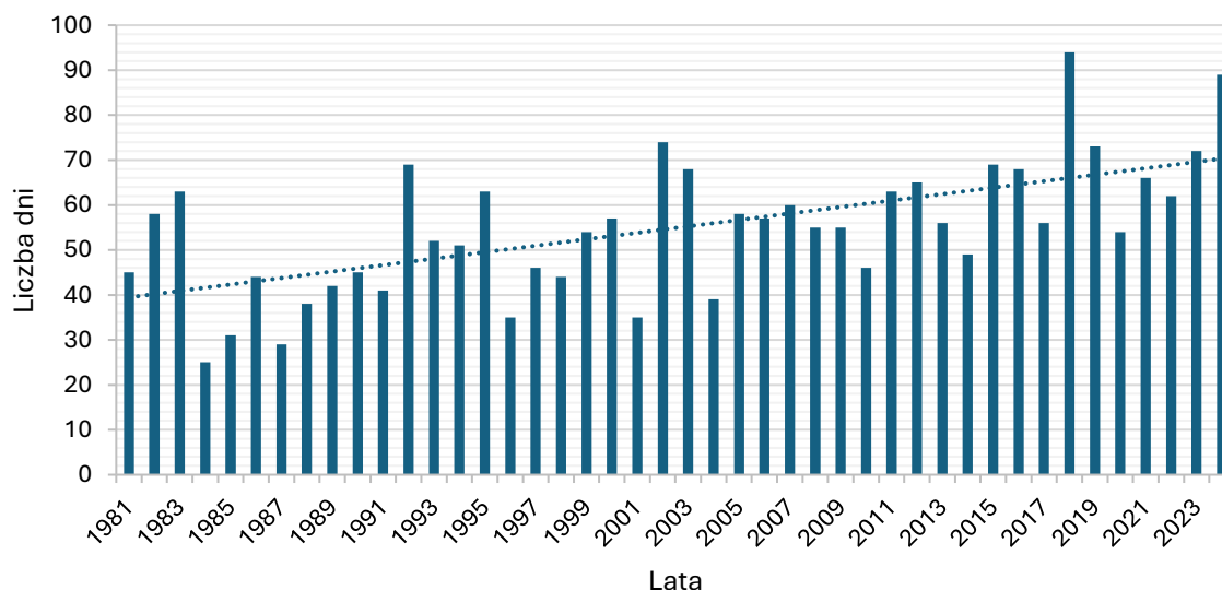
Wykres 5 Przebieg liczby dni gorących w Opolu 5
