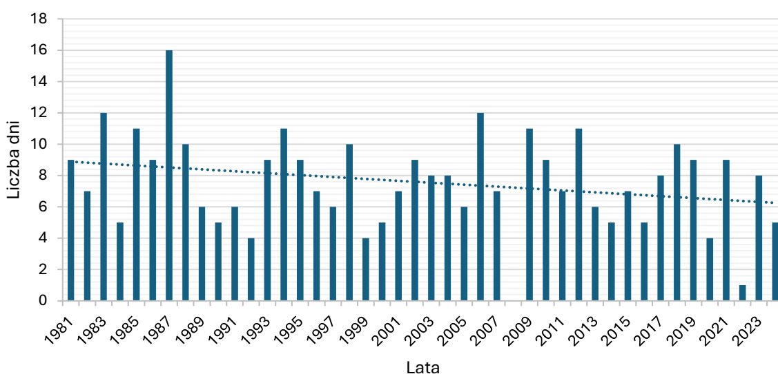
Wykres 12 Liczba dni z amplitudą dobową temperatury powietrza powyżej 6°C w Opolu 13
