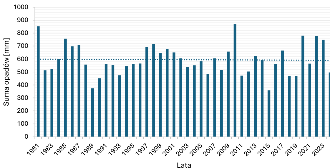
Wykres 15 Roczne sumy opadów w Opolu 16
