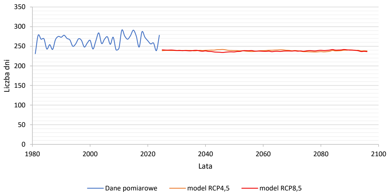
Wykres 11 Zmienność i prognozowane trendy zmian w liczbie dni bezopadowych w Opolu 15,16
