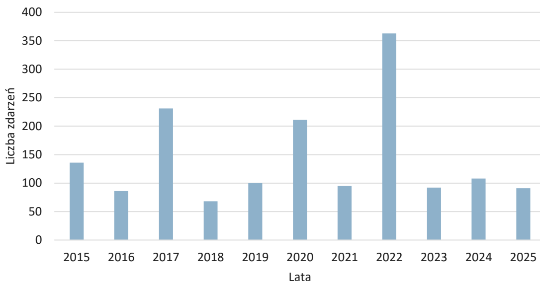
Rysunek 30 Liczba zdarzeń, interwencji podjętych przez w granicach Opola w wyniku występowania silnych wiatrów w latach 2015-2025 107
