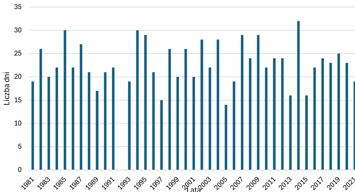
Wykres 30 Liczba dni w roku z burzą w Opolu 33
