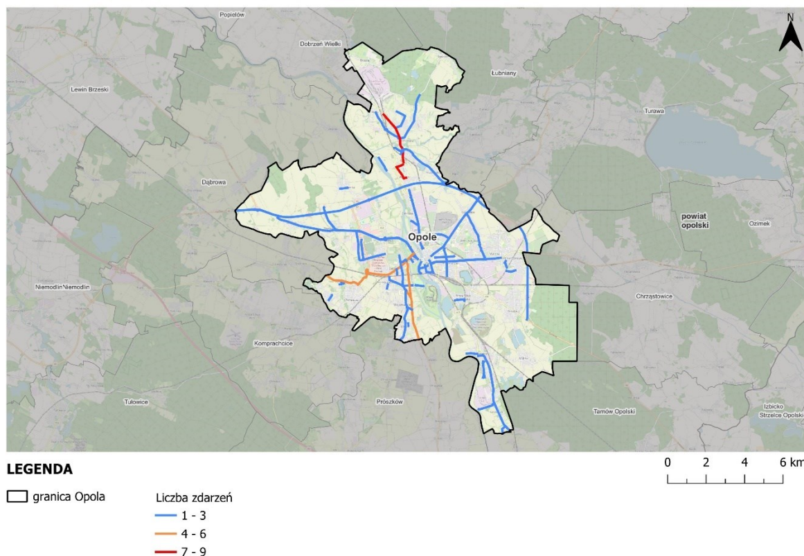
Rysunek 18 Lokalizacja zdarzeń, interwencji podjętych przez Państwową Straż Pożarną w granicach Opola w wyniku przyboru wód w latach 2015-2025 76
