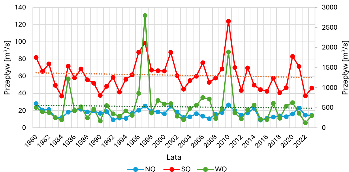
Wykres 27 Przebieg wartości NQ, SQ oraz WQ dla posterunku wodowskazowego Racibórz-Miedonia 29
