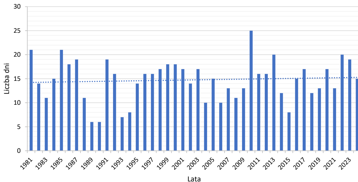
Wykres 3 Częstość występowania opadów atmosferycznych o sumie dobowej co najmniej 10 mm w Opolu 3
