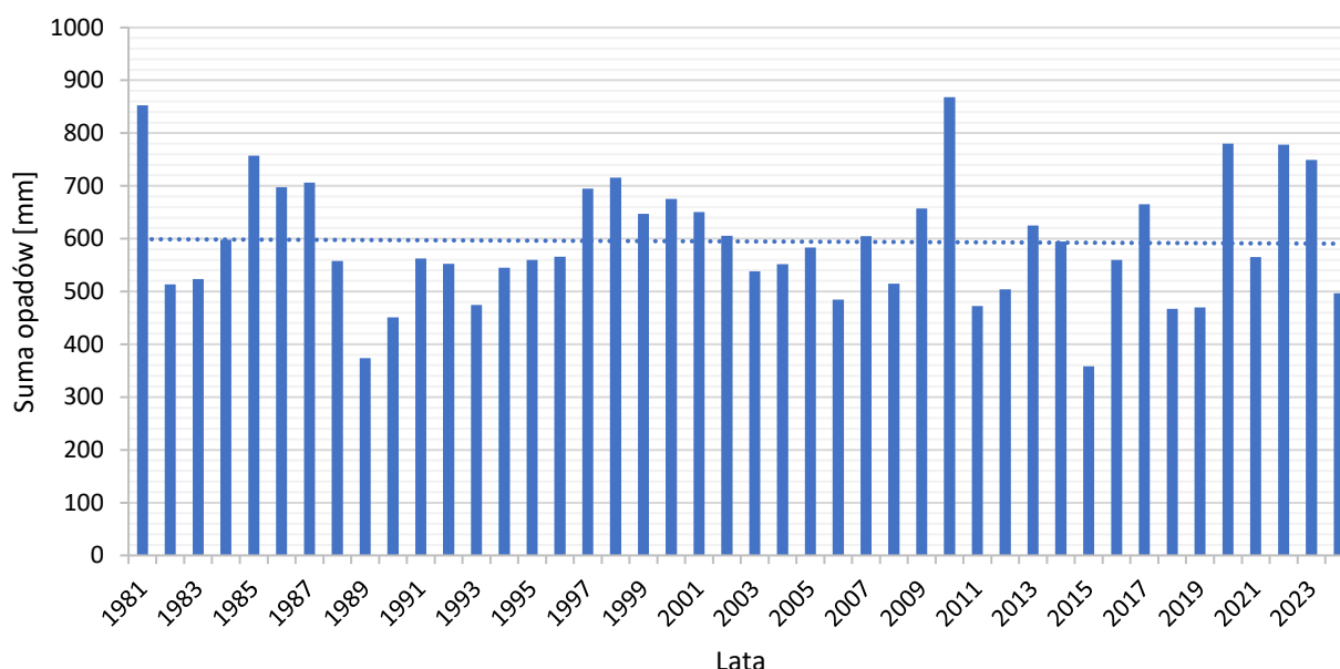
Wykres 1 Roczne sumy opadów w Opolu 1
