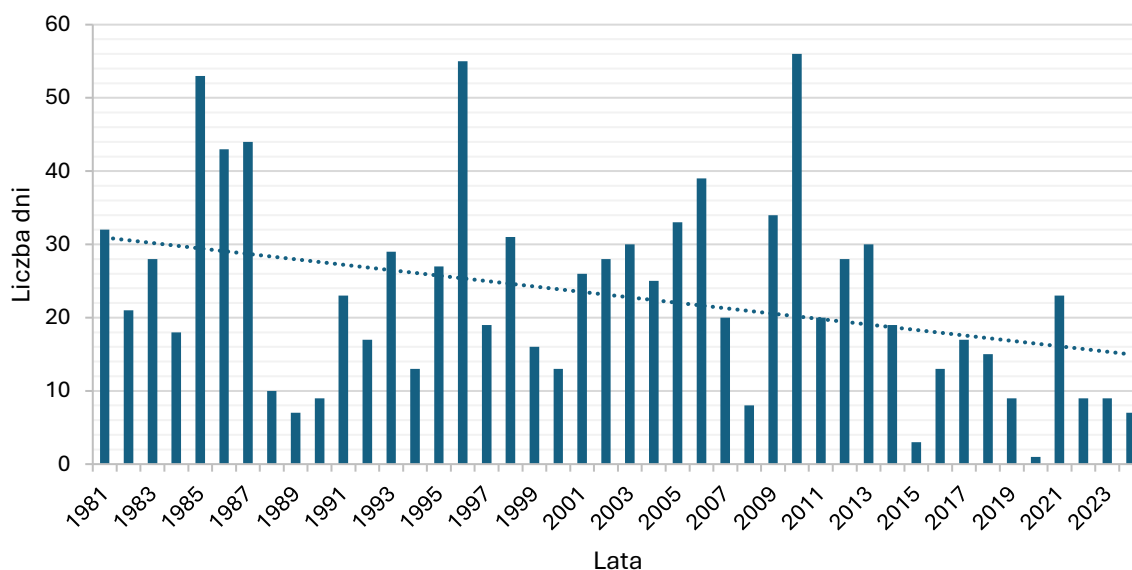
Wykres 8 Przebieg liczby dni mroźnych w Opolu 8
