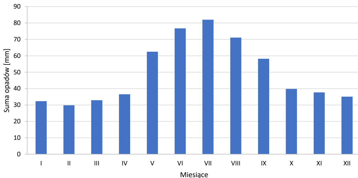
Wykres 2 Przebieg średnich miesięcznych sum opadów w Opolu 2
