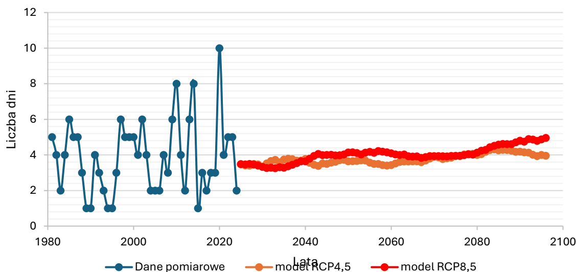
Wykres 36 Zmienność i prognozowane trendy zmian liczby dni w roku z opadami >20 mm w Opolu 57,58
