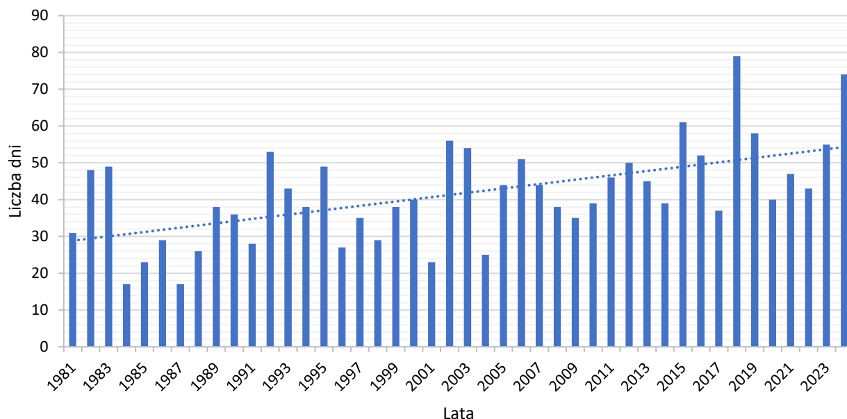
Wykres 6 Liczba dni bezopadowych z temperaturą maksymalną wyższą niż 25°C w Opolu 7
