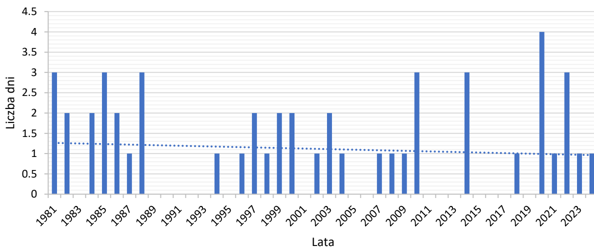
Wykres 5 Częstość występowania opadów atmosferycznych o sumie dobowej co najmniej 30 mm w Opolu 5
