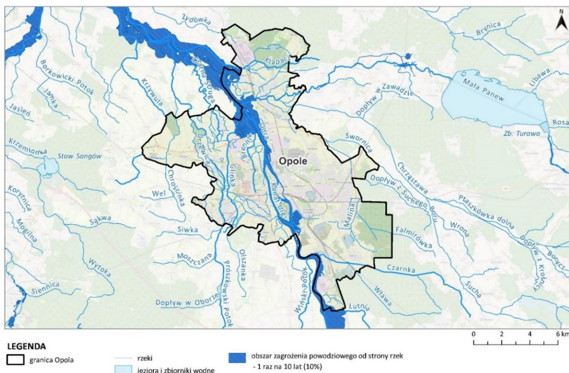
Rysunek 23 Obszary zagrożenia powodziowego 10% w zasięgu Opola 86
