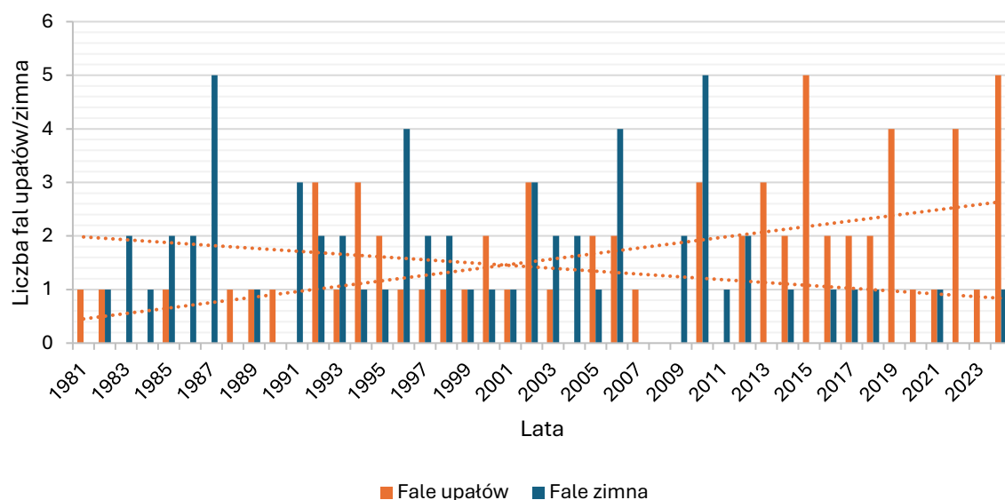
Wykres 10 Najdłuższy ciąg fal upałów i fal zimna w Opolu 11
