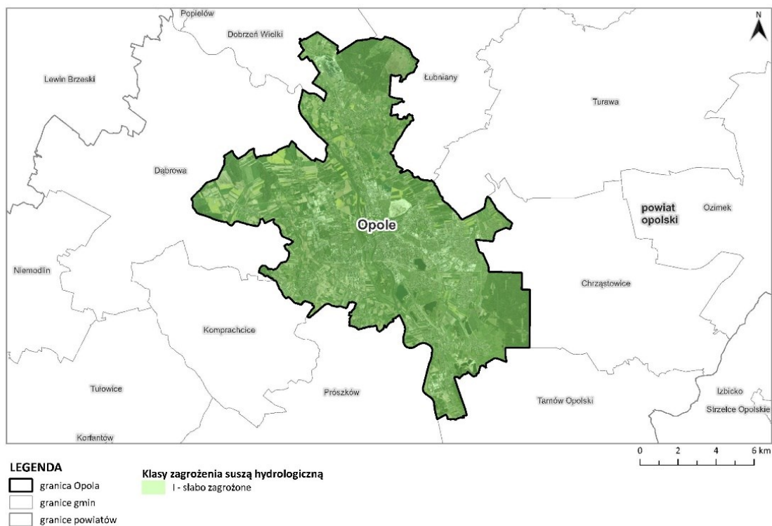
Rysunek 27 Zagrożenie suszą hydrologiczną w zasięgu Opola 93
