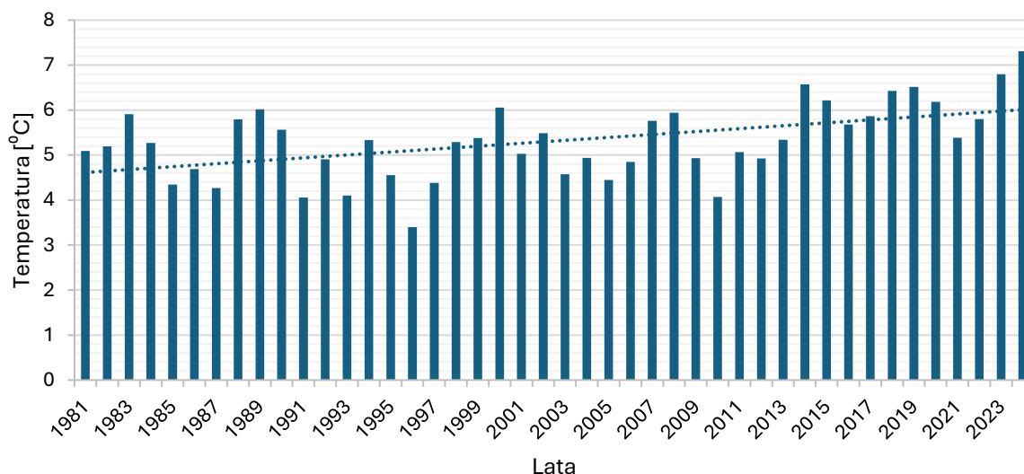
Wykres 4 Przebieg średnich dobowych wartości temperatury wraz z minimalną dobową powietrza w Opolu 4
