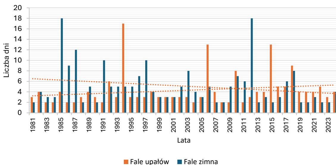
Wykres 9 Liczba przypadków fal upałów i zimna w Opolu 10
