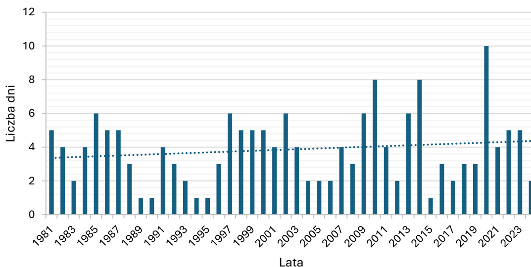
Wykres 18 Częstość występowania opadów atmosferycznych o sumie dobowej co najmniej 20 mm w Opolu 19
