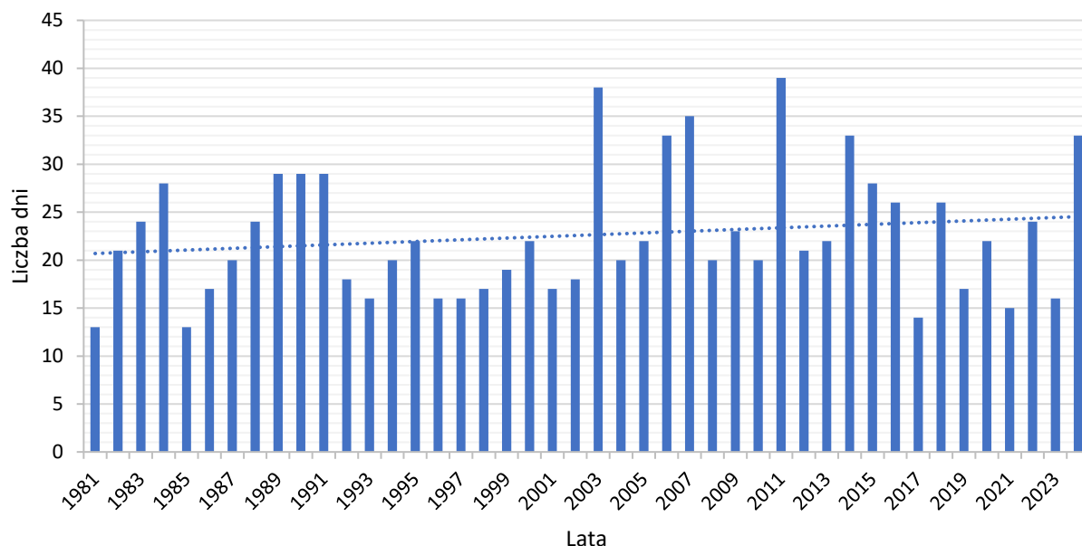
Wykres 7 Najdłuższy ciąg dni bez opadu w Opolu 8
