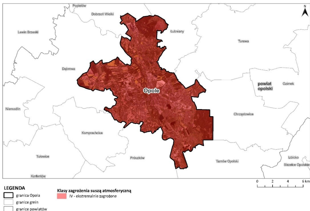
Rysunek 25 Zagrożenie suszą atmosferyczną w zasięgu Opola 91
