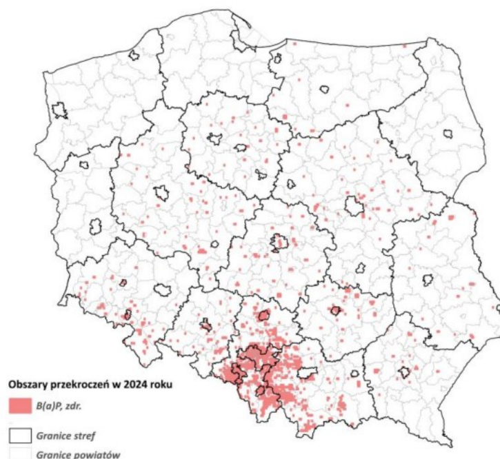
Rysunek 1 Zasięgi obszaru przekroczenia oszacowanego dla średniego rocznego stężenia benzo(a)pirenu w pyłe zawieszonym PM10 na obszarze Polski w 2024 roku 36
