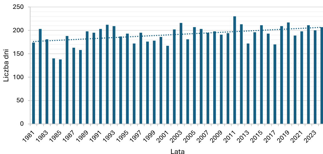
Wykres 11 Liczba dni z amplitudą dobową temperatury powietrza powyżej 8°C w Opolu 12
