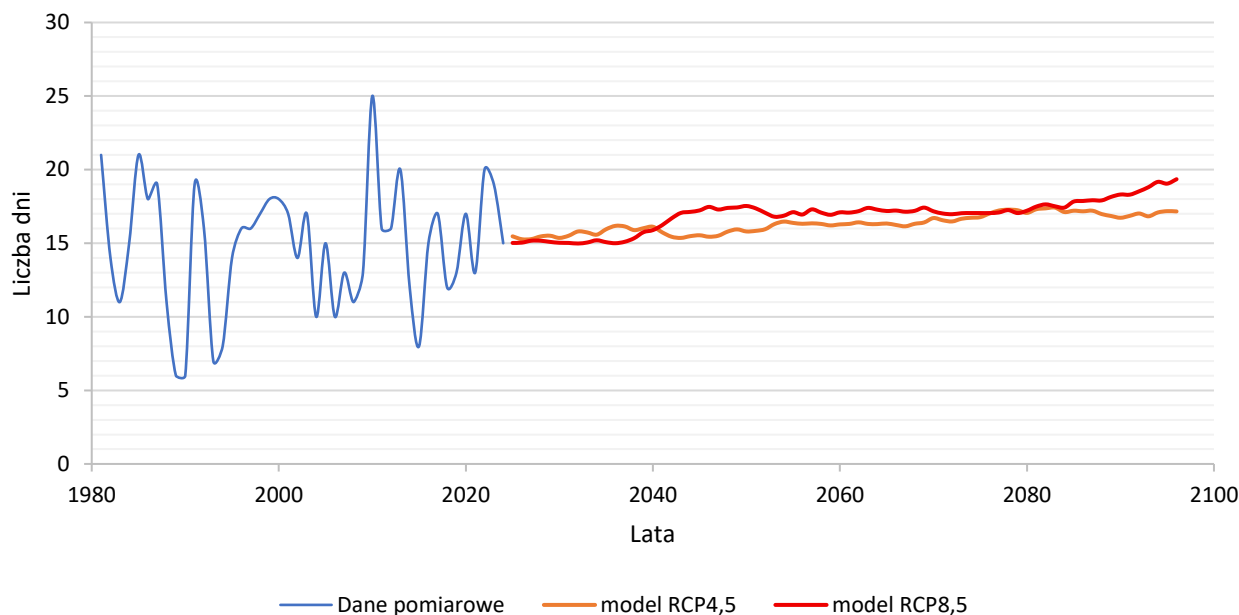
Wykres 9 Zmienność i prognozowane trendy zmian liczby dni w roku z opadami >10 mm w Opolu 11,12
