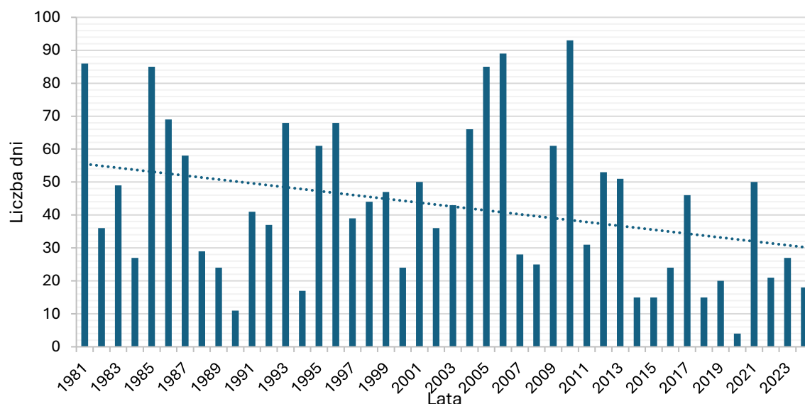
Wykres 22 Częstość występowania pokrywy śnieżnej w Opolu 24
