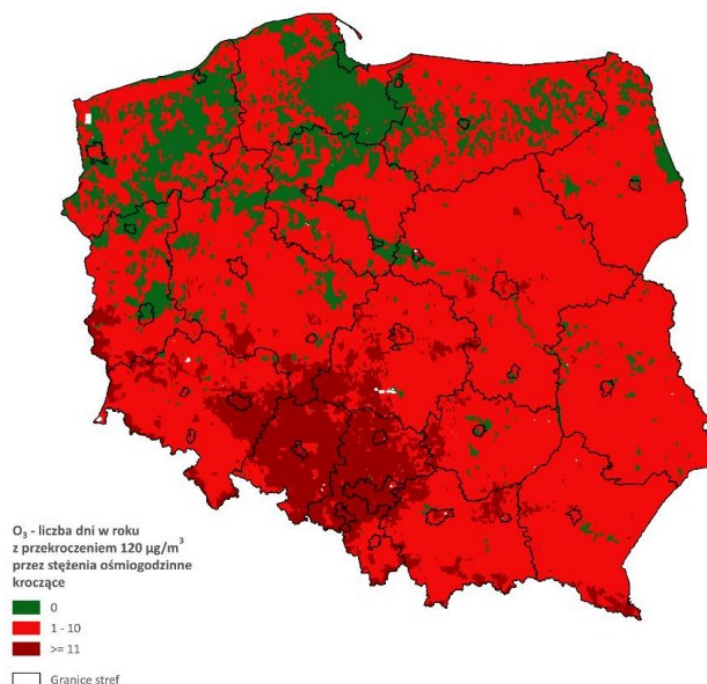
Rysunek 4. Rozkład przestrzenny stężenia O 3 na obszarze Polski w 2024 roku, wyrażony jako liczba dni w roku z przekroczeniem poziomu 120 µg/m 3 przez wartości średnie 8-godzinne kroczące, określony na podstawie modelowania matematycznego oraz obiektywnego szacowania 46
