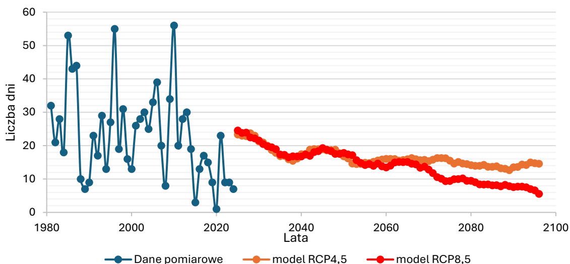
Wykres 33 Zmienność i prognozowane trendy zmian liczby dni mroźnych w Opolu 51,52
