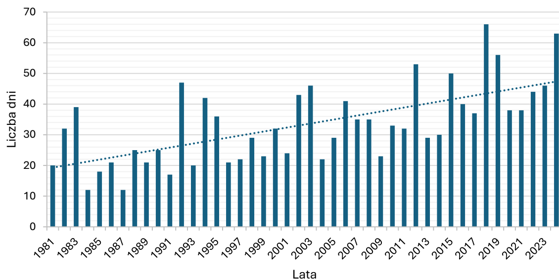
Wykres 14 Liczba dni z CDD>27 dla sezonu letniego w Opolu 15
