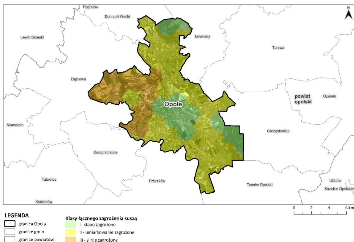
Rysunek 29. Łączne zagrożenie suszą w zasięgu Opola 96
