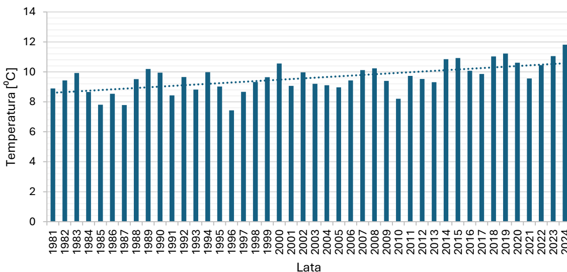
Wykres 1 Wieloletnia zmienność średniej rocznej temperatury powietrza w Opolu, wraz z linią trendu 1
