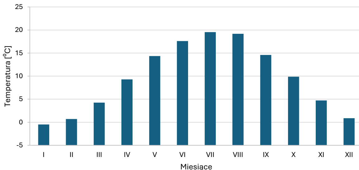
Wykres 2 Przebieg roczny średniej miesięcznej temperatury powietrza w Opolu 2
