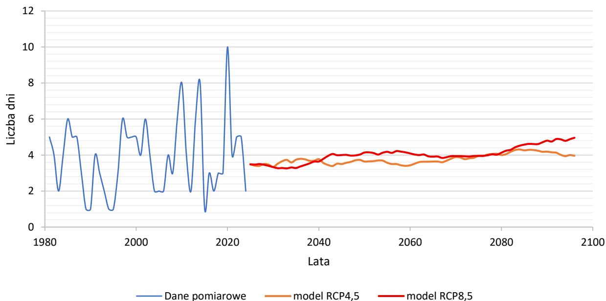
Wykres 10 Zmienność i prognozowane trendy zmian liczby dni w roku z opadami >20 mm w Opolu 13,14
