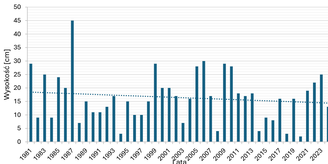
Wykres 24 Maksymalna wysokość pokrywy śnieżnej w Opolu 26
