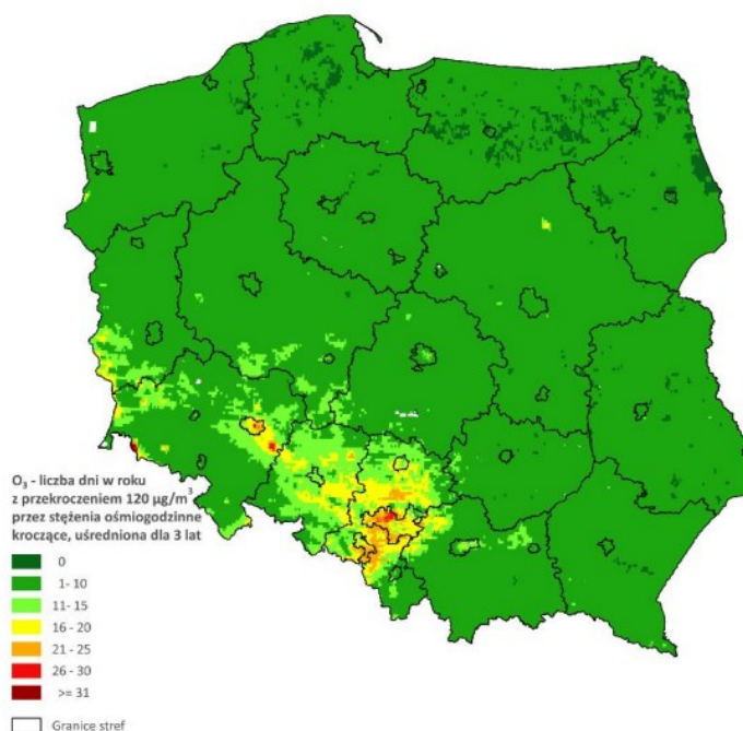
Rysunek 3. Rozkład przestrzenny stężenia O 3 na obszarze Polski w 2024 roku, wyrażony jako liczba dni w roku z przekroczeniem poziomu 120 µg/m 3 przez wartości średnie 8-godzinne kroczące, uśredniona dla 3 lat, określony na podstawie modelowania matematycznego 44
