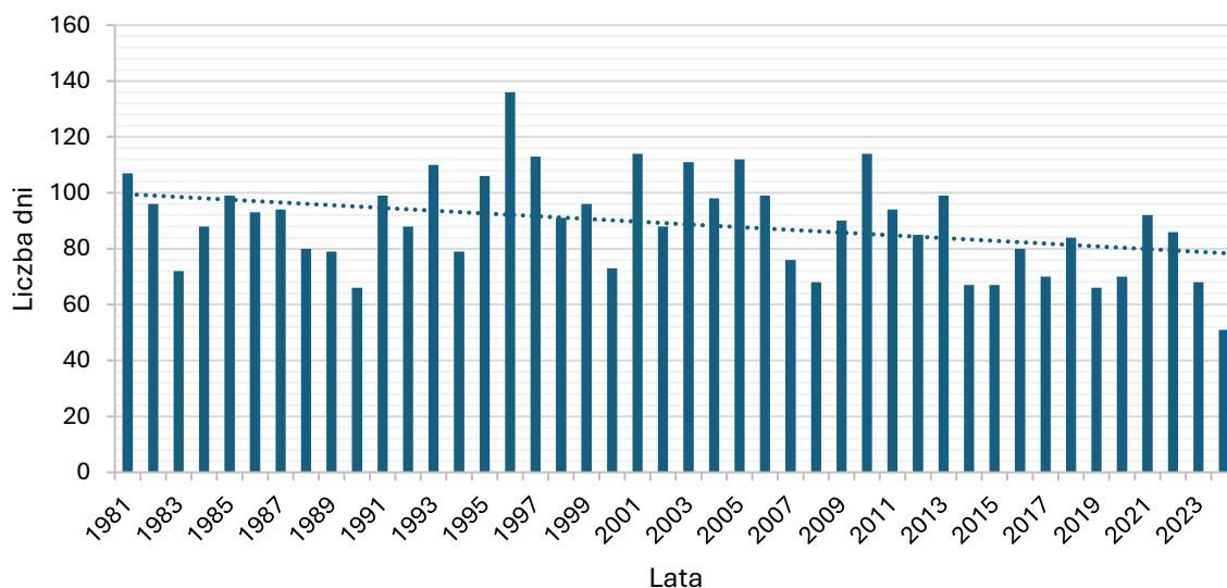
Wykres 7 Przebieg liczby dni przymrozkowych w Opolu 7
