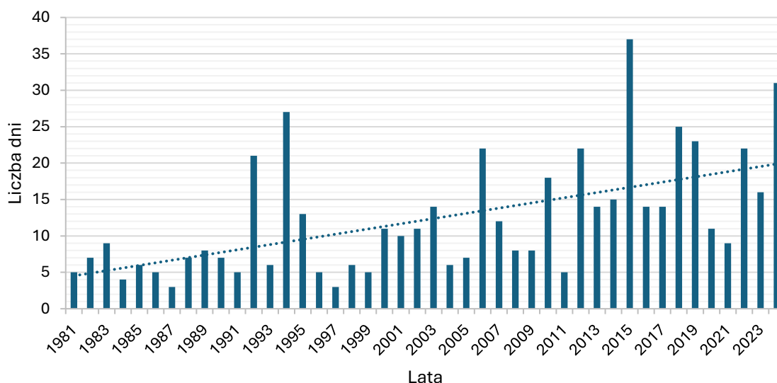
Wykres 6 Przebieg liczby dni upalnych w Opolu 6
