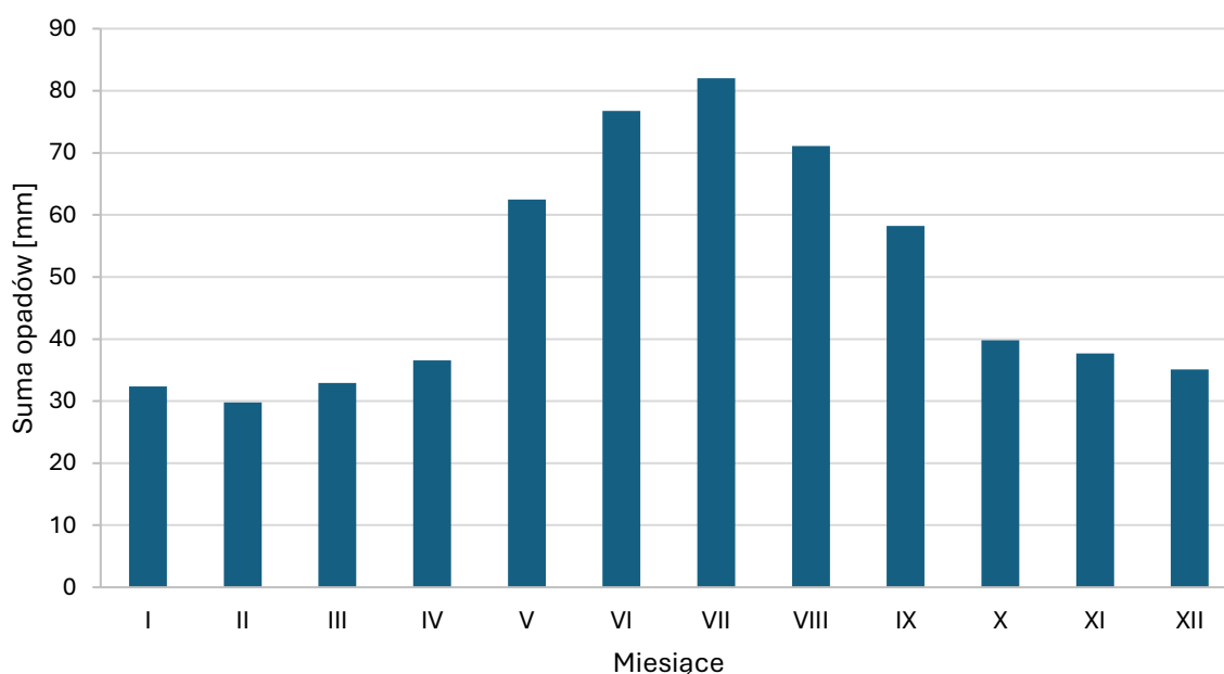
Wykres 16 Przebieg średnich miesięcznych sum opadów w Opolu 17
