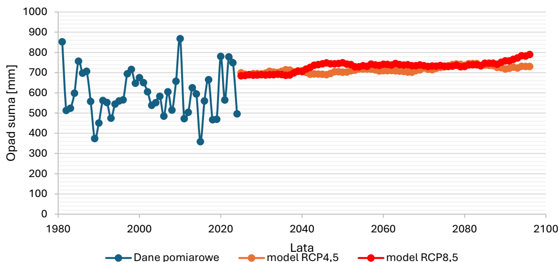
Wykres 34 Zmienność i prognozowane trendy zmian rocznym sum opadów atmosferycznych w Opolu 53,54
