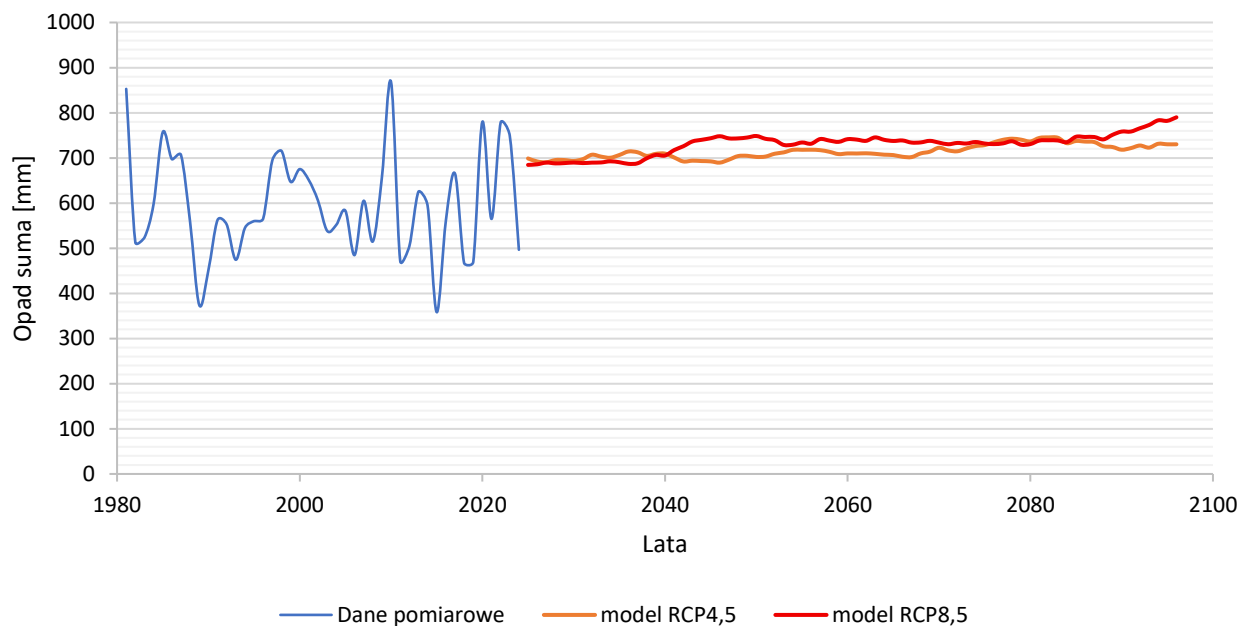
Wykres 8 Zmienność i prognozowane trendy zmian rocznych sum opadów atmosferycznych w Opolu 9,10
