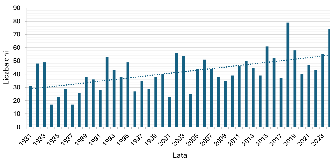
Wykres 20 Liczba dni bezopadowych z temperaturą maksymalną wyższą niż 25°C w Opolu 22
