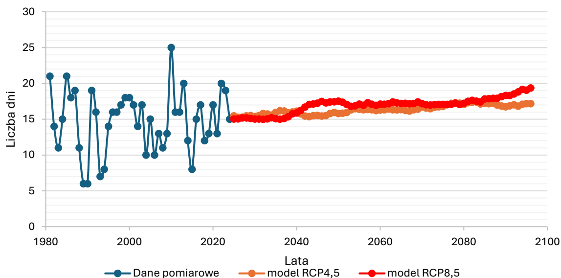
Wykres 35 Zmienność i prognozowane trendy zmian liczby dni w roku z opadami >10 mm w Opolu 55,56
