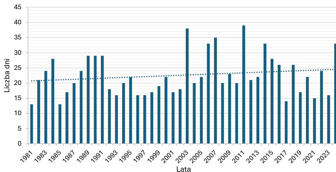
Wykres 21 Najdłuższy ciąg dni bez opadu w Opolu 23
