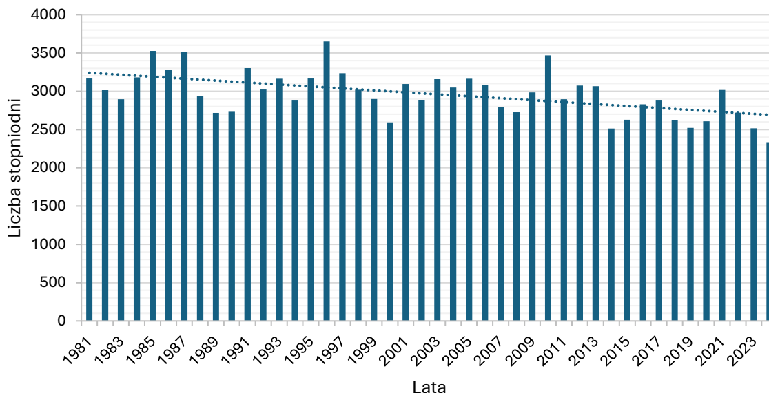
Wykres 13 Liczba stopniodni HDD<17 w Opolu 14
