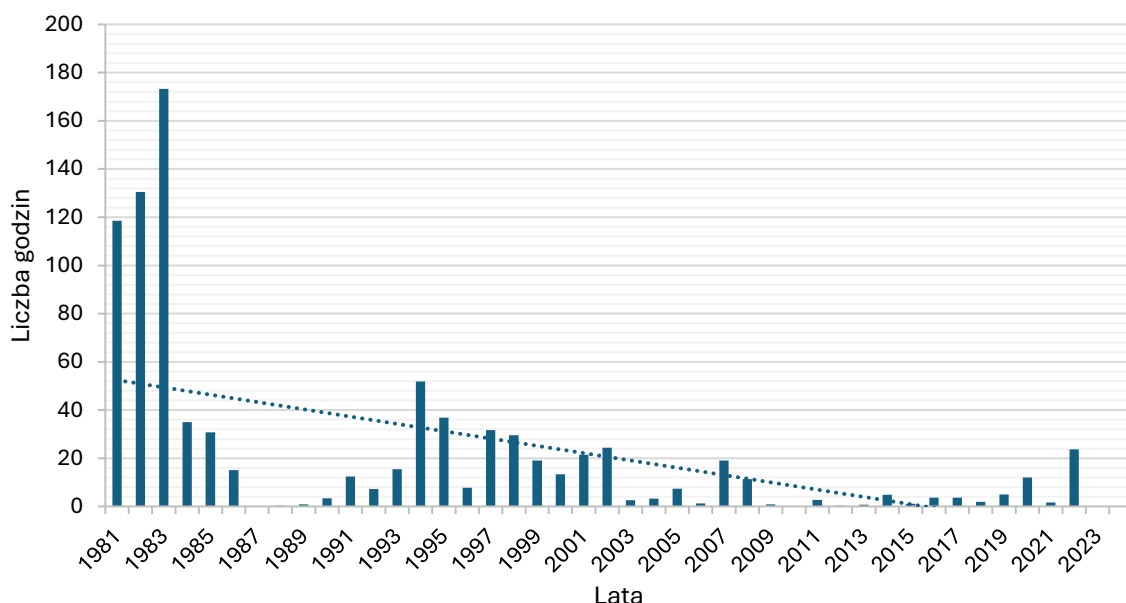
Wykres 29 Liczba godzin w roku trwania wiatru \geq 10 \text{ m/s} w Opolu 32
