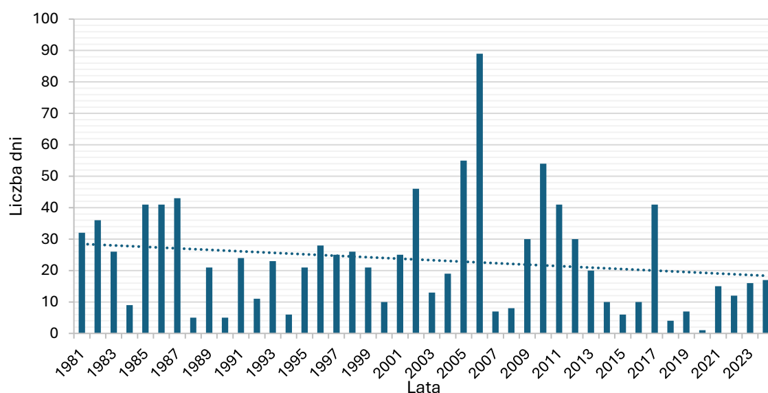
Wykres 23 Najdłuższy ciąg dni z pokrywą śnieżną w Opolu 25
