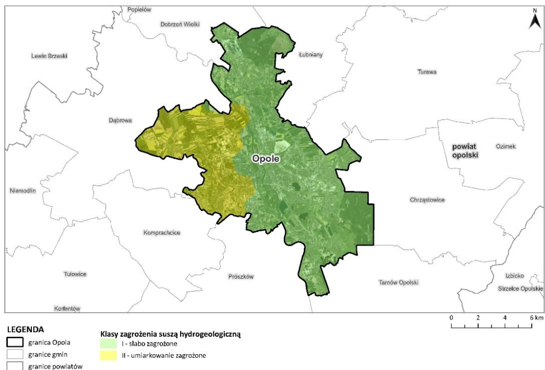
Rysunek 28 Zagrożenie suszą hydrogeologiczną w zasięgu Opola 94
